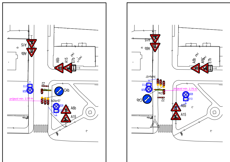
Typizovaný překop obousměrné vozovky po polovinách
