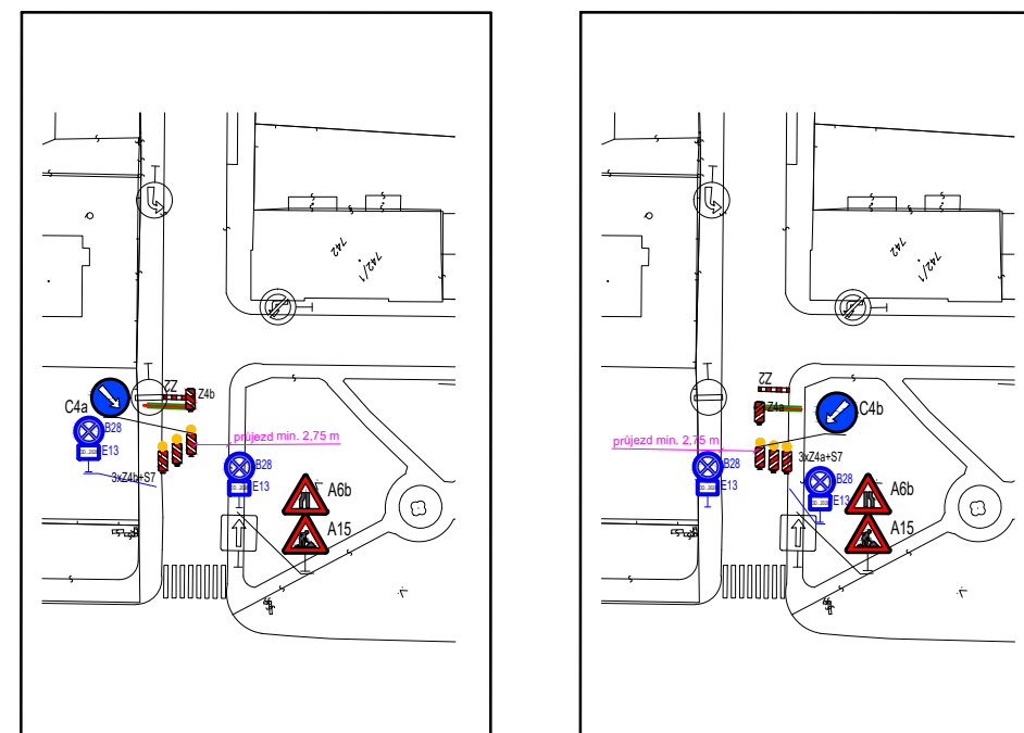
Typizovaný překop jednosměrné vozovky po polovinách
